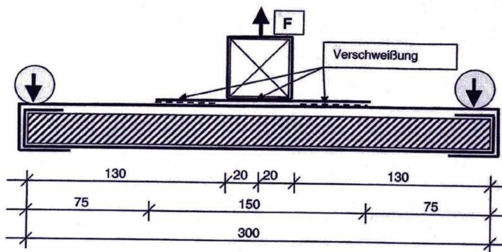
Figura 2: Campione della serie V14, sezione, misurazioni in mm
