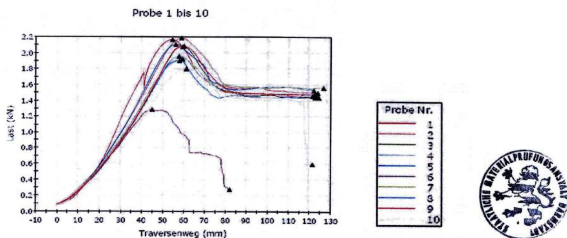
Figura 4: Diagramma di formatura della forza, Serie V13, FPO, Produttore 5
